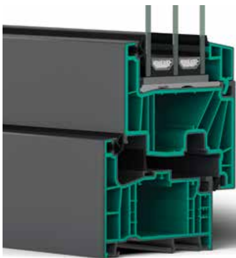
Recyklované materiály v jádru profilu ARTEVO a v zasklívacích lištách
